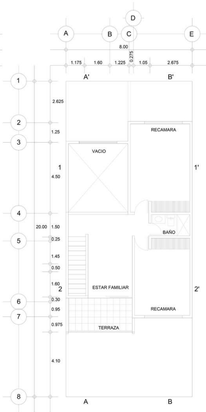
PLANTA ARQUITECTONICA (P.A.)
