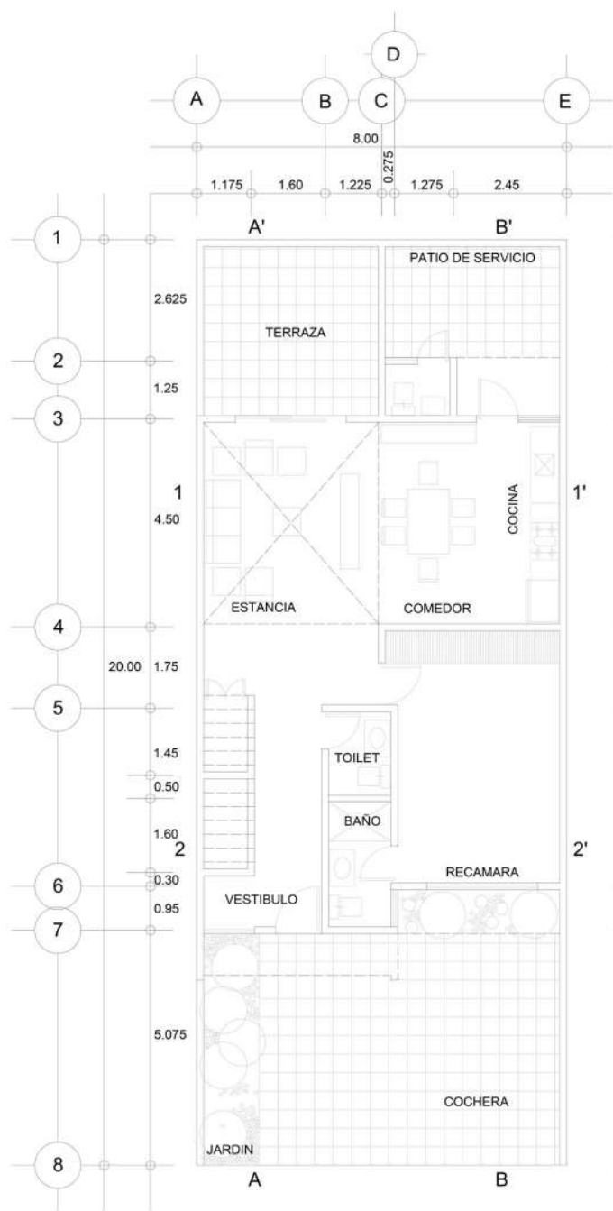
PLANTA ARQUITECTONICA (P.B.)
