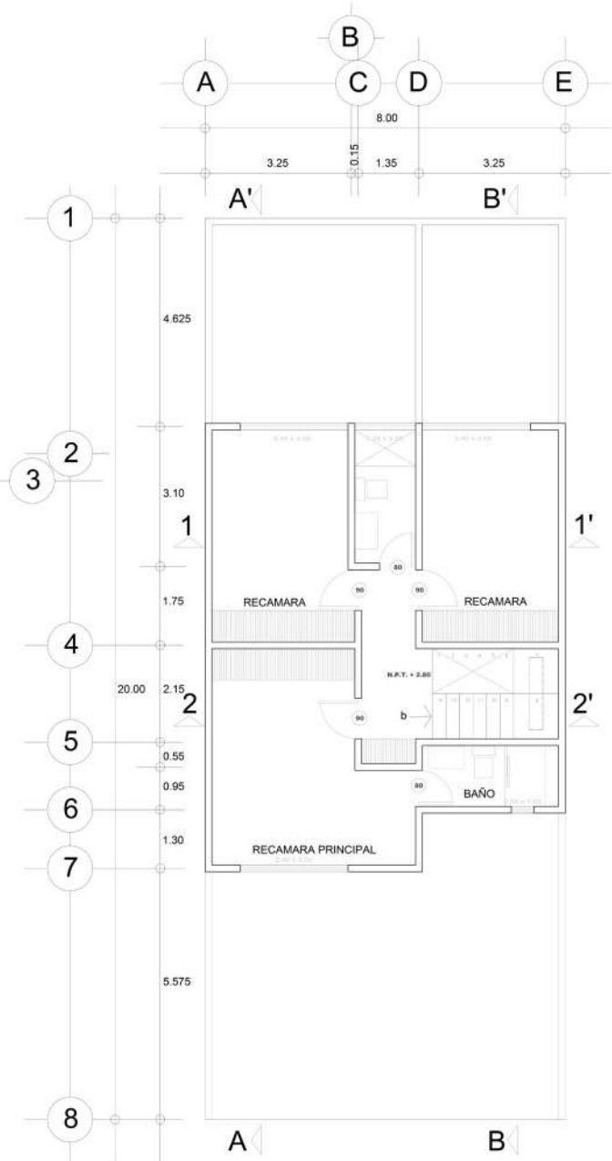
PLANTA ARQUITECTONICA P.A. ESCALA 1:75
